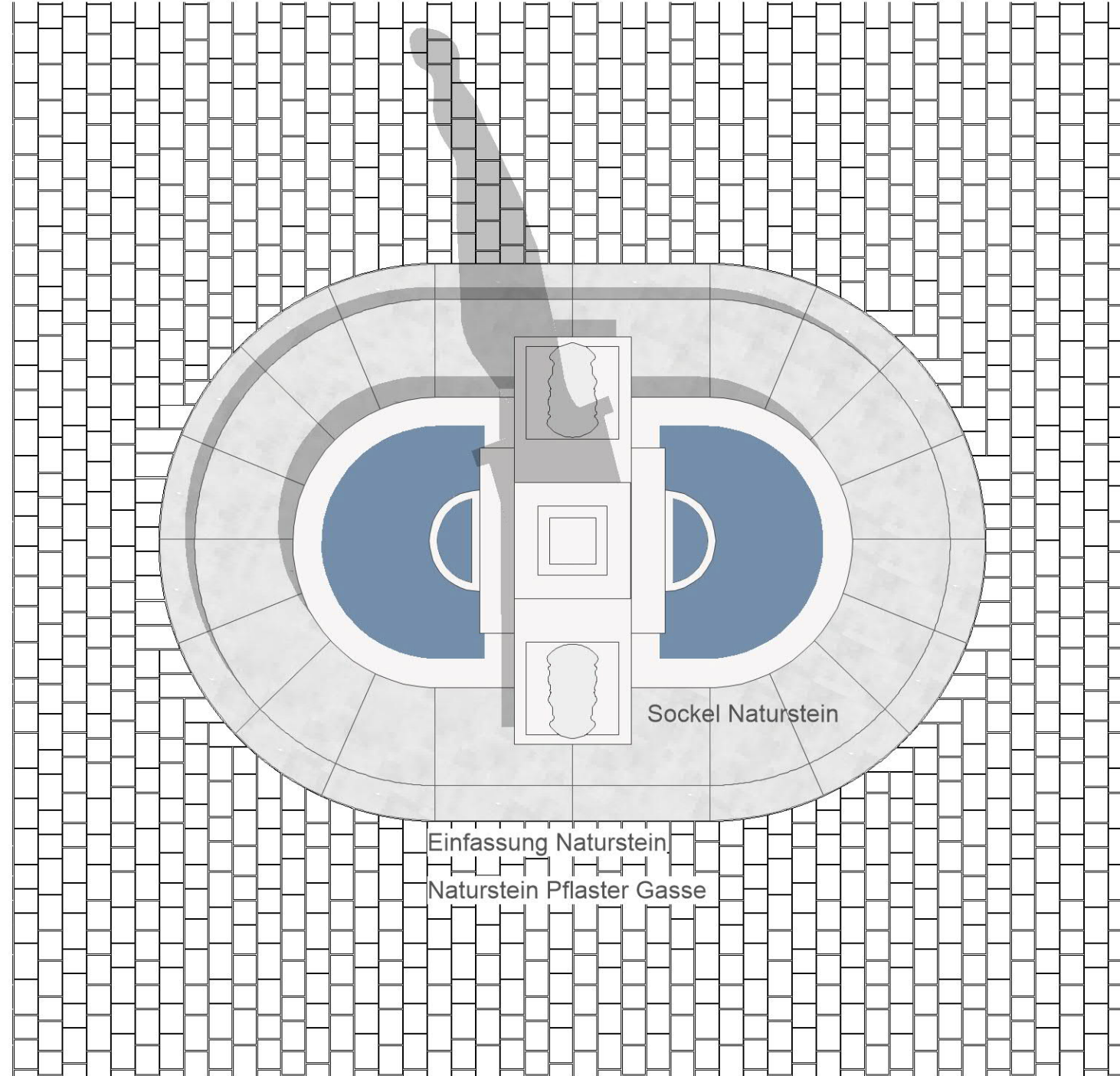
Aufsicht 1:50
