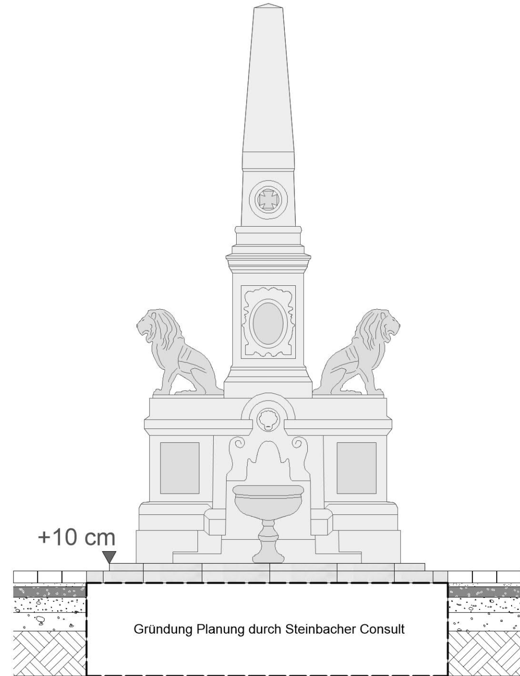
Schnitt 1:50
